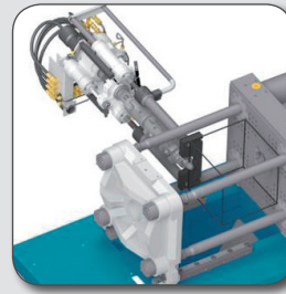
Horizontale oder vertikale Befestigung der Spritzaggregate an der Werkzeugseite (L – Position)
