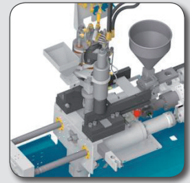
Spritzaggregat in verschiebbarer Position auf der festen Platte
