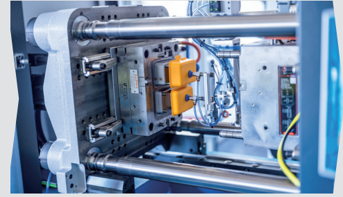
Synchronisierung der Bewegungen von LR 5 und elektrischem Auswerfer
