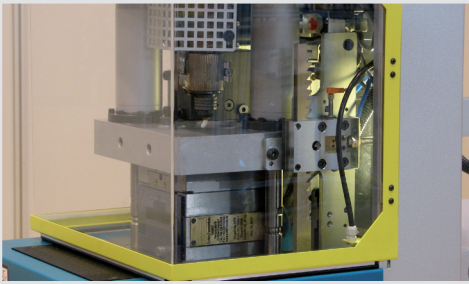
Diagonal angeordnete Holme ermöglichen eine bessere Zugänglichkeit
