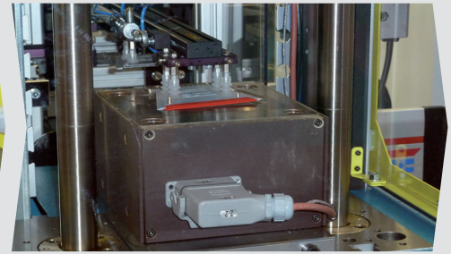
Automatisierte Zuführung/Entnahme der Einlegeteile vom hinteren Maschinentisch
