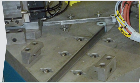
Manueller Schiebetisch (auf Anfrage) (z. B. mit Linear- oder Y-Führung)
